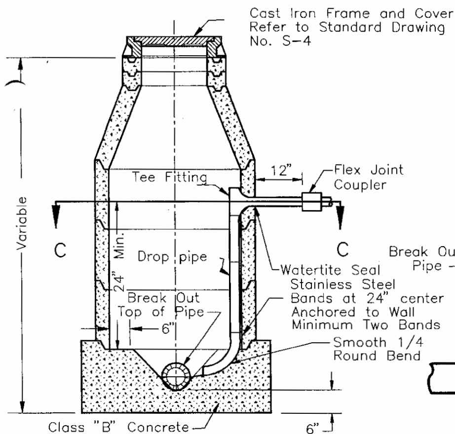
SECTION A-A
